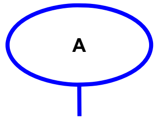
Attribut
