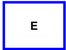
Entity-Menge
