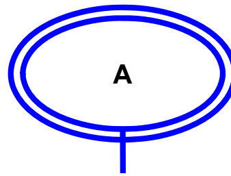
mehrwertiges Attribut
