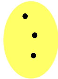
VORLESUNGSTEILNAHME
