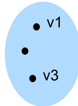
VORLESUNG
