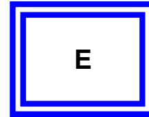
schwache Entity-Menge
