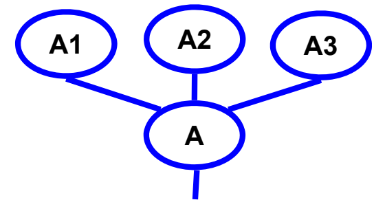
zusammengesetztes Attribut
